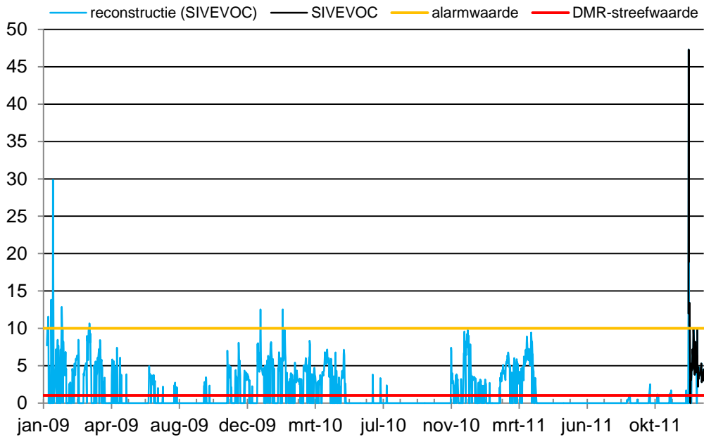
Figuur 17: Aceton in de Maas bij Eijsden [ \mu\text{g/l} ]
