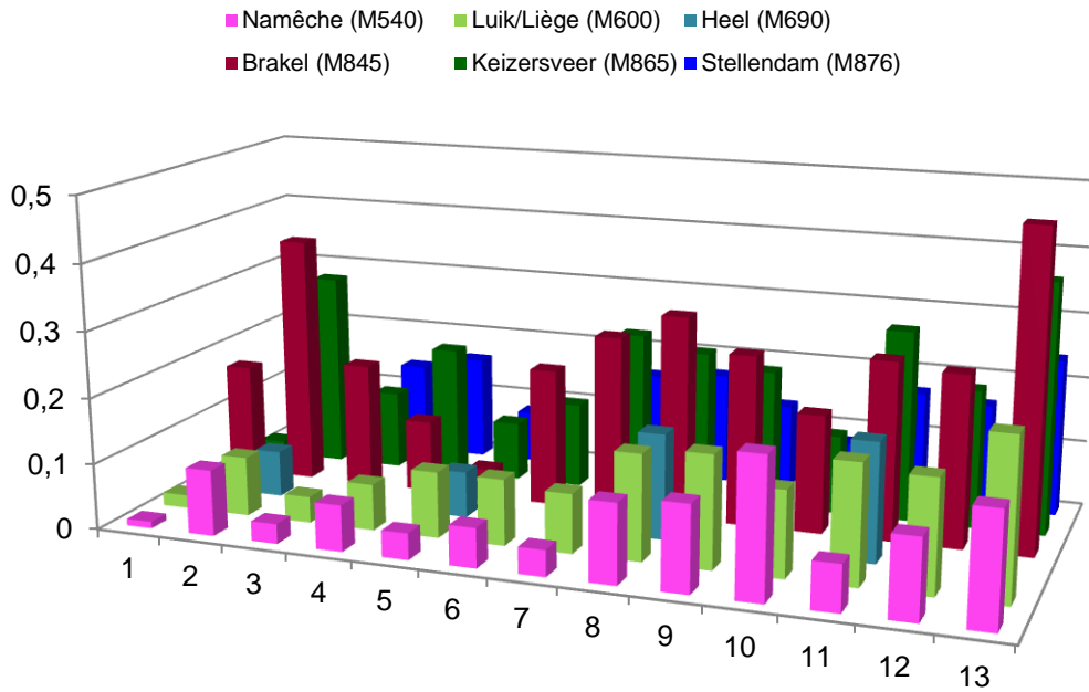
Figuur 10: Amidotrizoïnezuur in de Maas in 2011 [ \mu\text{g/l} ]
