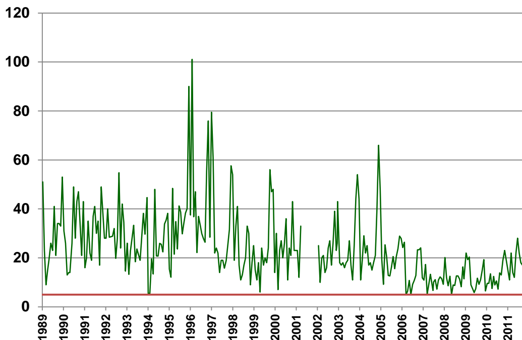
Figuur 14: EDTA in de Maas bij Keizersveer 1989-2011 [ \mu\text{g/l} ]
